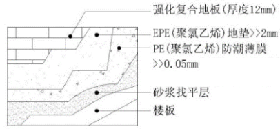
地板悬浮式安装节点
