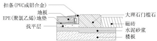
扣条施工节点图
