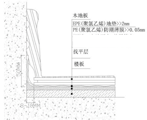
踢脚板与地板相接处剖面图
